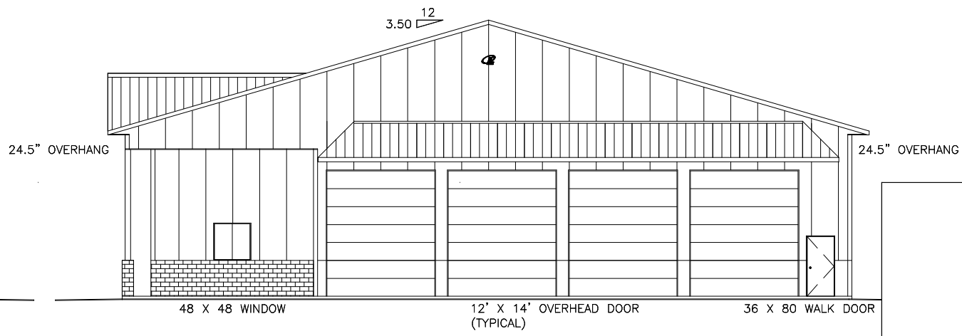
D16 ENDWALL #2 ELEVATION SCALE: 1/16=1
